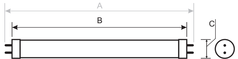
A: 1213mm B:1198mm C:Φ26mm
